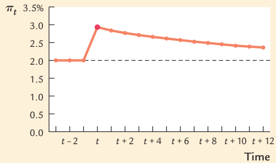
(d) Inflation
